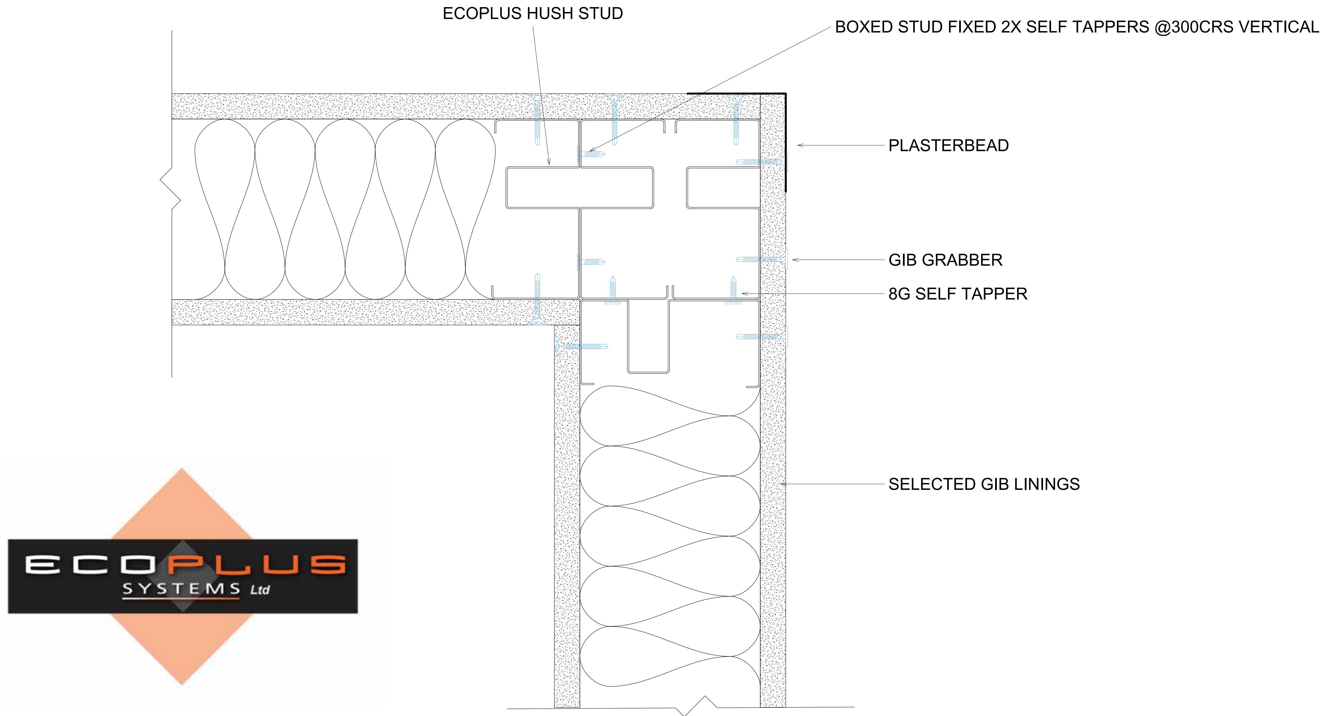
External Corner - ECOPLUS HUSH STUD
